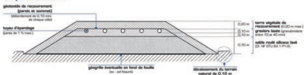
coupe transversale
