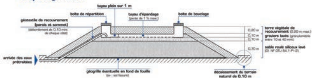
coupe longitudinale
