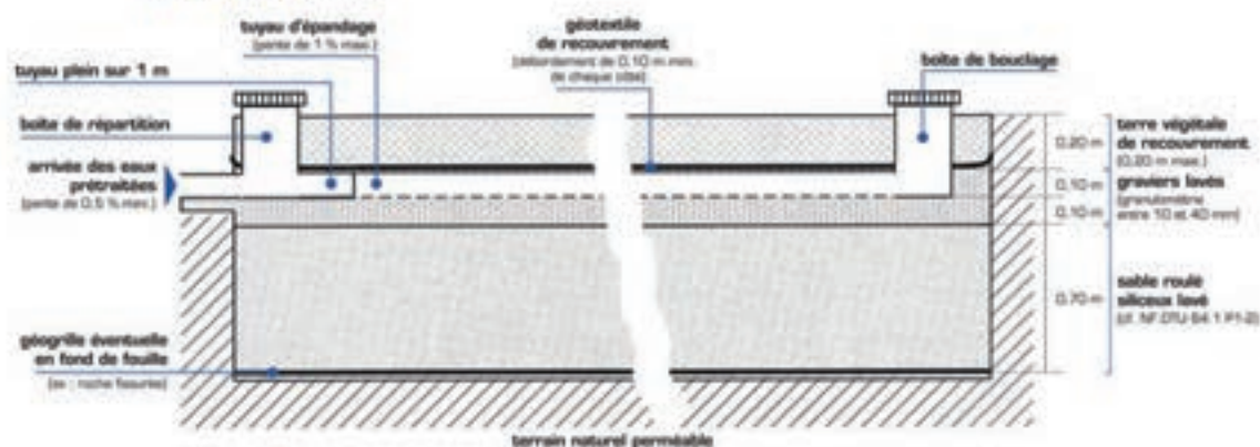
coupe longitudinale
