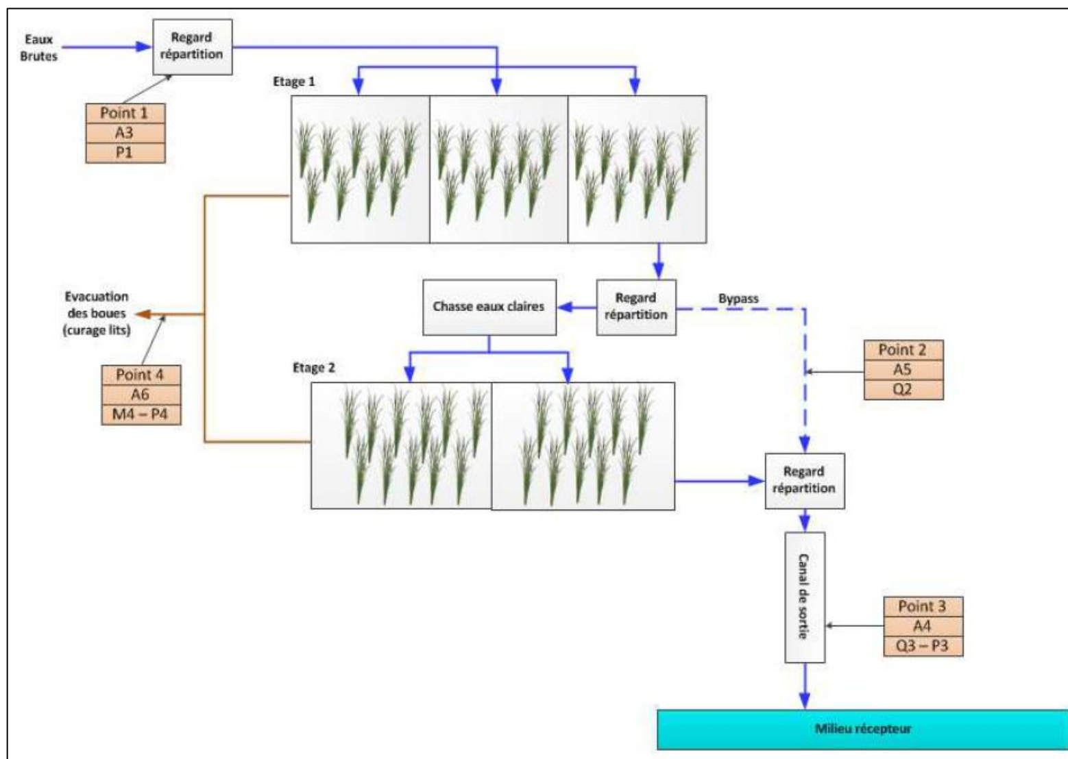
Figure 15 : Synoptique des ouvrages de traitement – STEP Suzette (Source : CDV)
