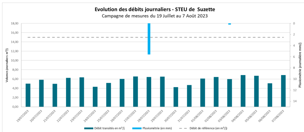
Figure 17: Evolution des débits journaliers estivaux – Entrée de STEU de Suzette- Campagne été 2023
