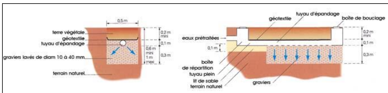
Figure 23 : Schéma d'une tranchée d'infiltration (source : Landru.fr)
