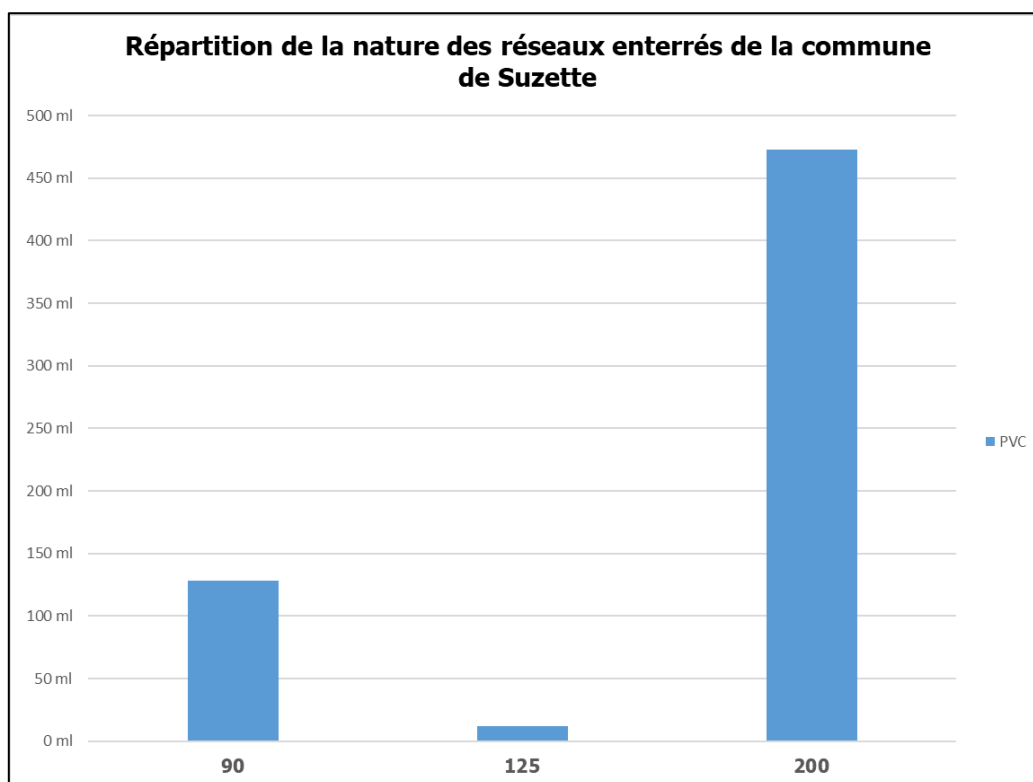
Figure 12 : Répartition des réseaux d'eaux usées de Suzette en fonction des matériaux et diamètres
