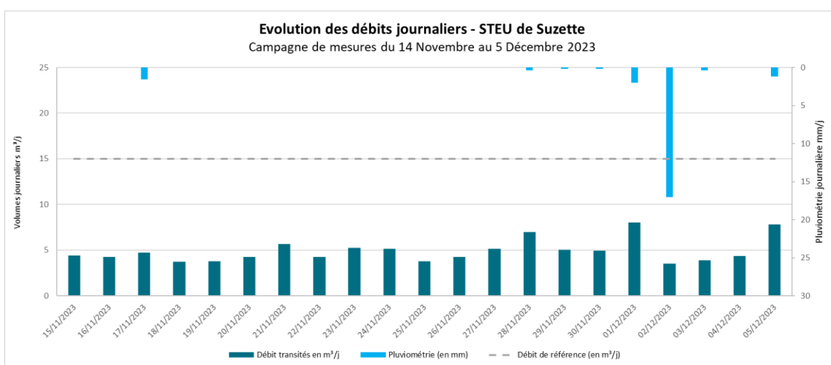
Figure 18: Evolution des débits journaliers hivernaux – Entrée de STEU Suzette – Campagne hiver 2023
