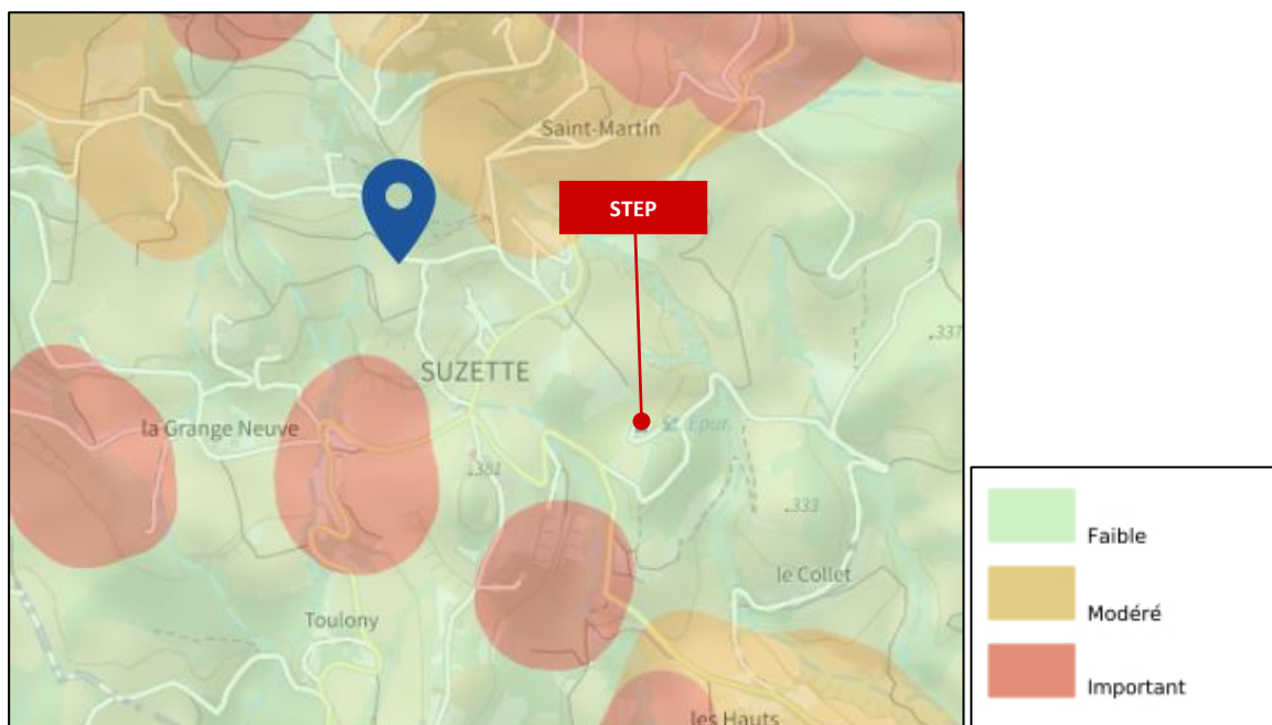
Figure 7 : Cartographie des aléas retrait-gonflement des argiles sur Suzette (Géorisques)
