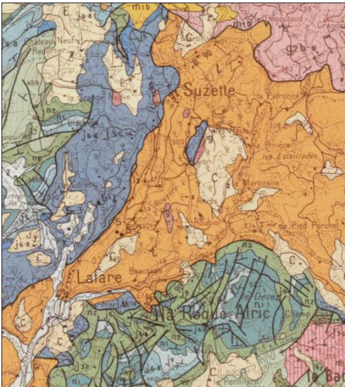
Figure 6 : Carte géologique du secteur (source : Infoterre)
